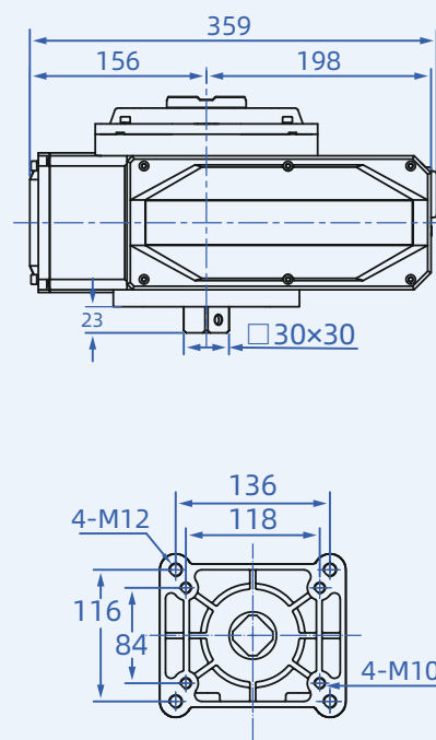
标准式
