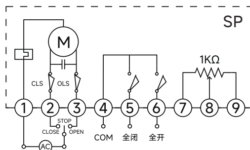
H型
