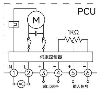
PCU型
