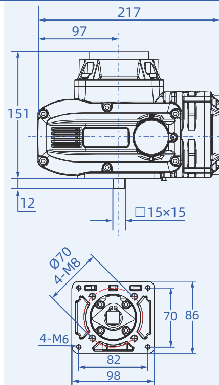
标准式
