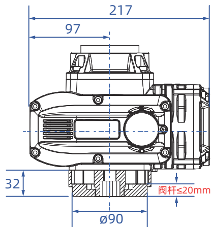
直装式
