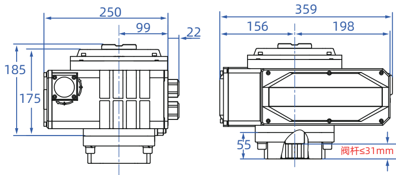
直装式
