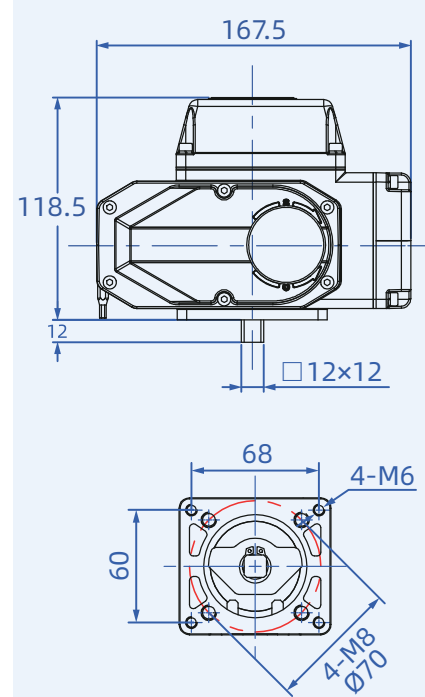
标准式
