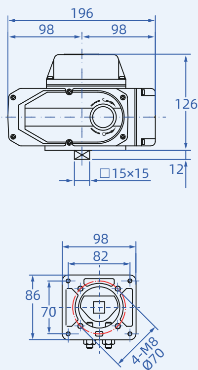
标准式
