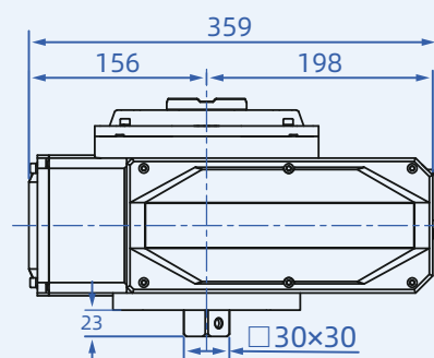
标准式
