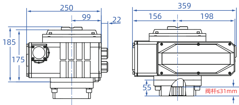
直装式
