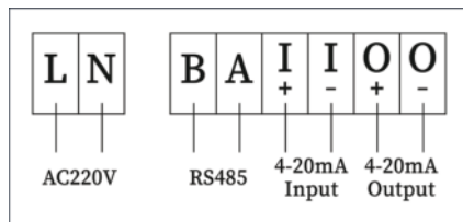
物联网微型执行器-AC220V
