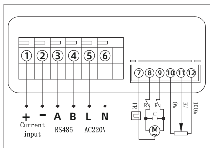
数字模块-AC-电路图
