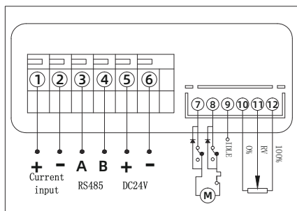
数字模块-DC-电路图
