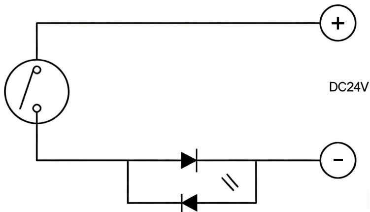
直流电磁阀接线图
