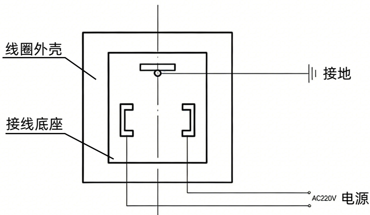
交流电磁阀接线图
